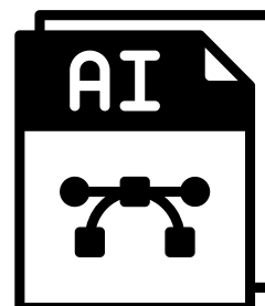
Ai Tools
